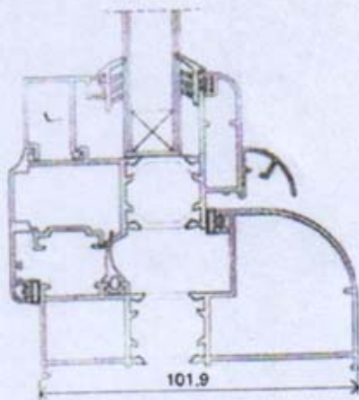
PRESEK 1-1
